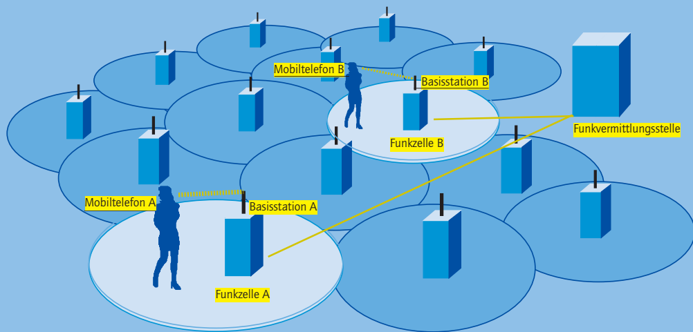
Struktur eines Mobilfunknetzes
